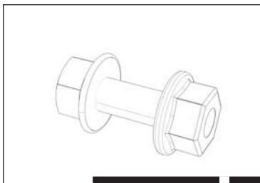
M6 - Schraube / Mutter DIN 692112 / 12 mm DIN 934 A2 M6
